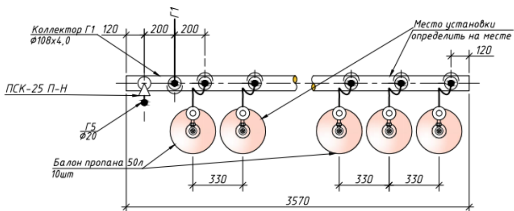
Рис.2. Рампа пропановая. Вид сверху.
