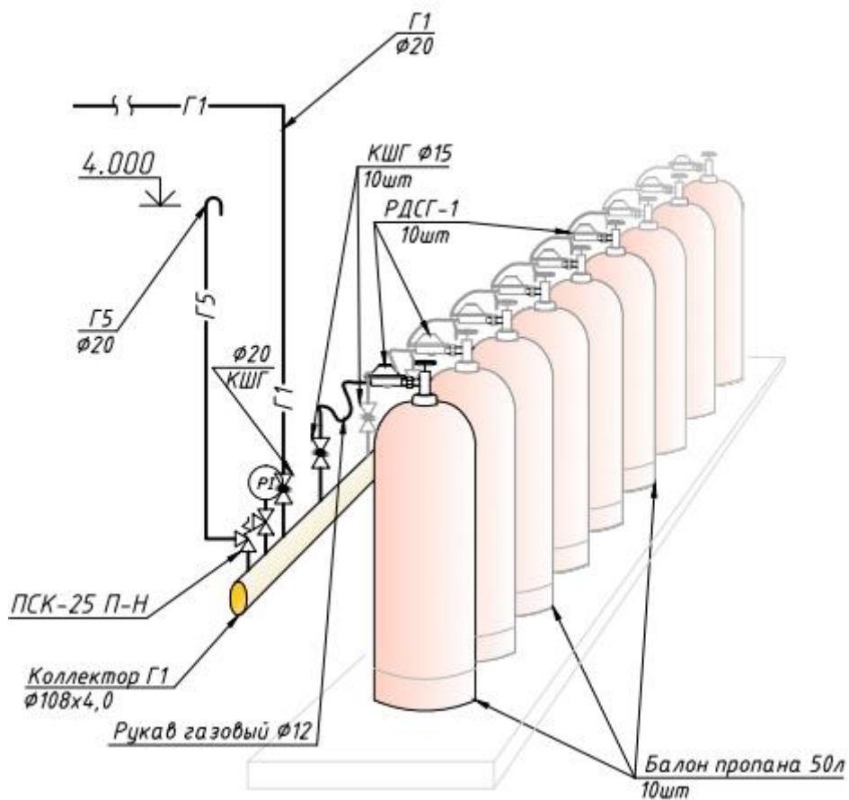
Рис.3. Рампа пропановая. Вид сбоку.
