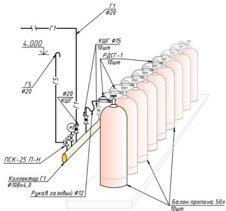
Рис.3. Рампа пропановая. Вид 2.
